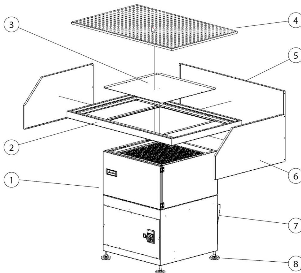
Abb. 2: Montage
