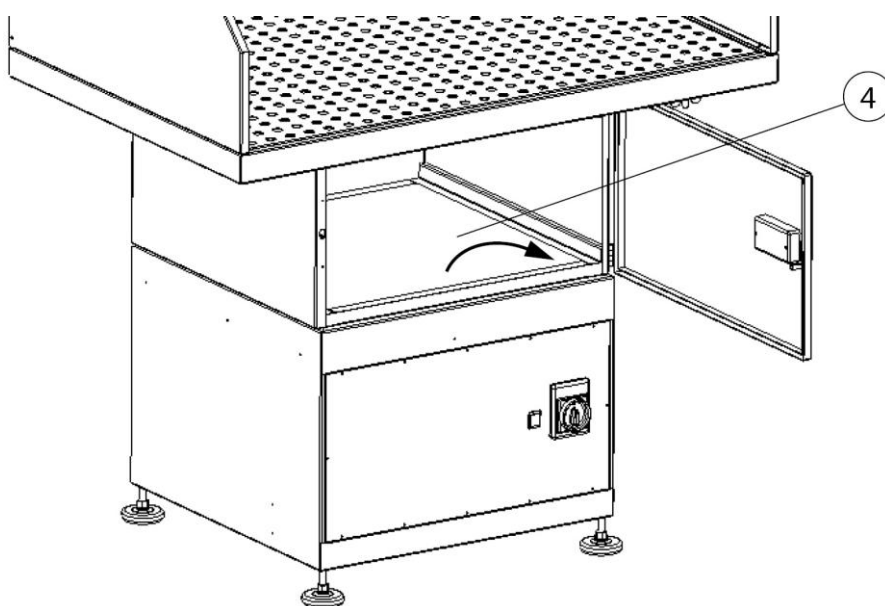
Abb. 11: Filterwechsel - Aktivkohlefilter (optional)
