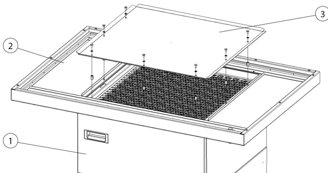
Abb. 3: Montage Luftleitblech + Schweißbrenner
